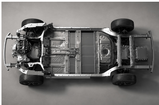
AWD de dois motores de alto desempenho
