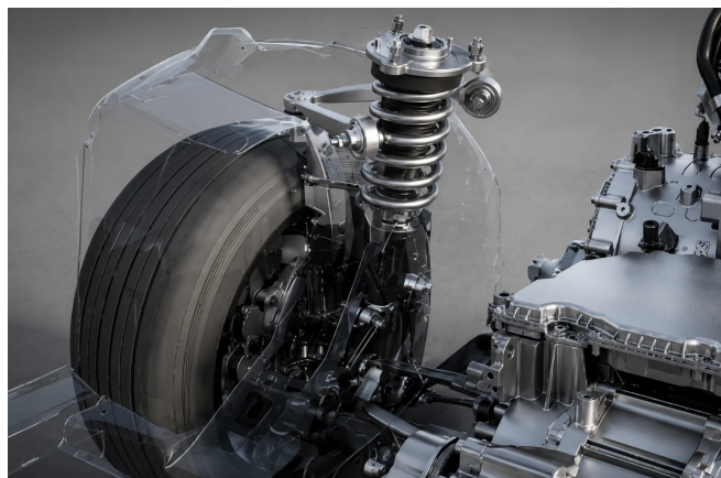
Duplo braço triangular dianteiro + suspensão traseira de braço em H Multi link
